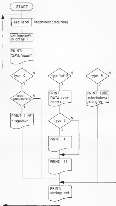
Afb. 6-5 Flowchart van het BASIC-programma 'labelprint'
